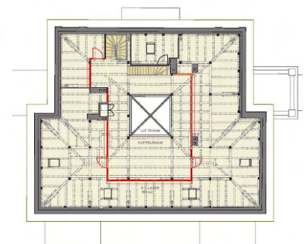
Dachgeschoss
